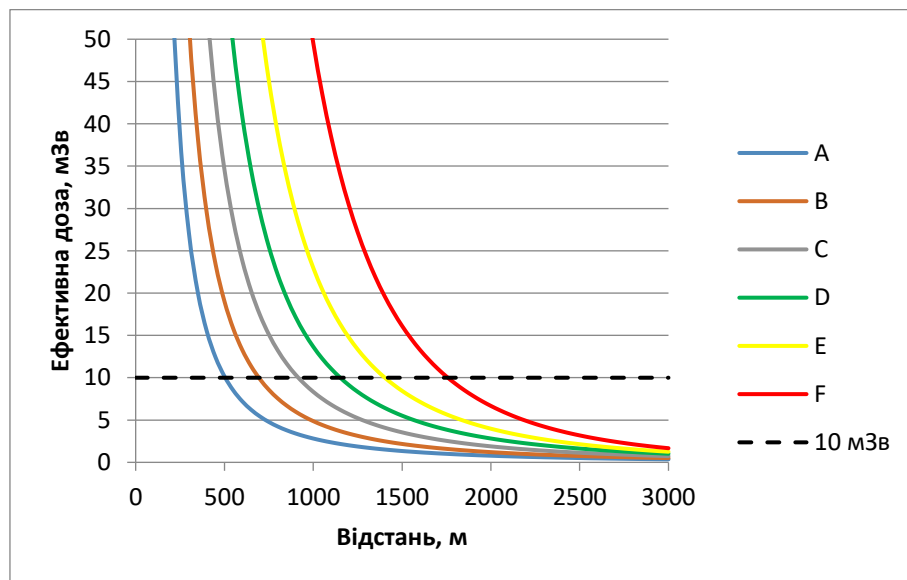
Рисунок 8.2– Залежність розрахункового значення ефективного дозування референтного віку «10 років» від відстані для різних категорій стійкості атмосфери Горизонтальною лінією позначено дозовий норматив 10 мЗв для дітей при проєктних аваріях
