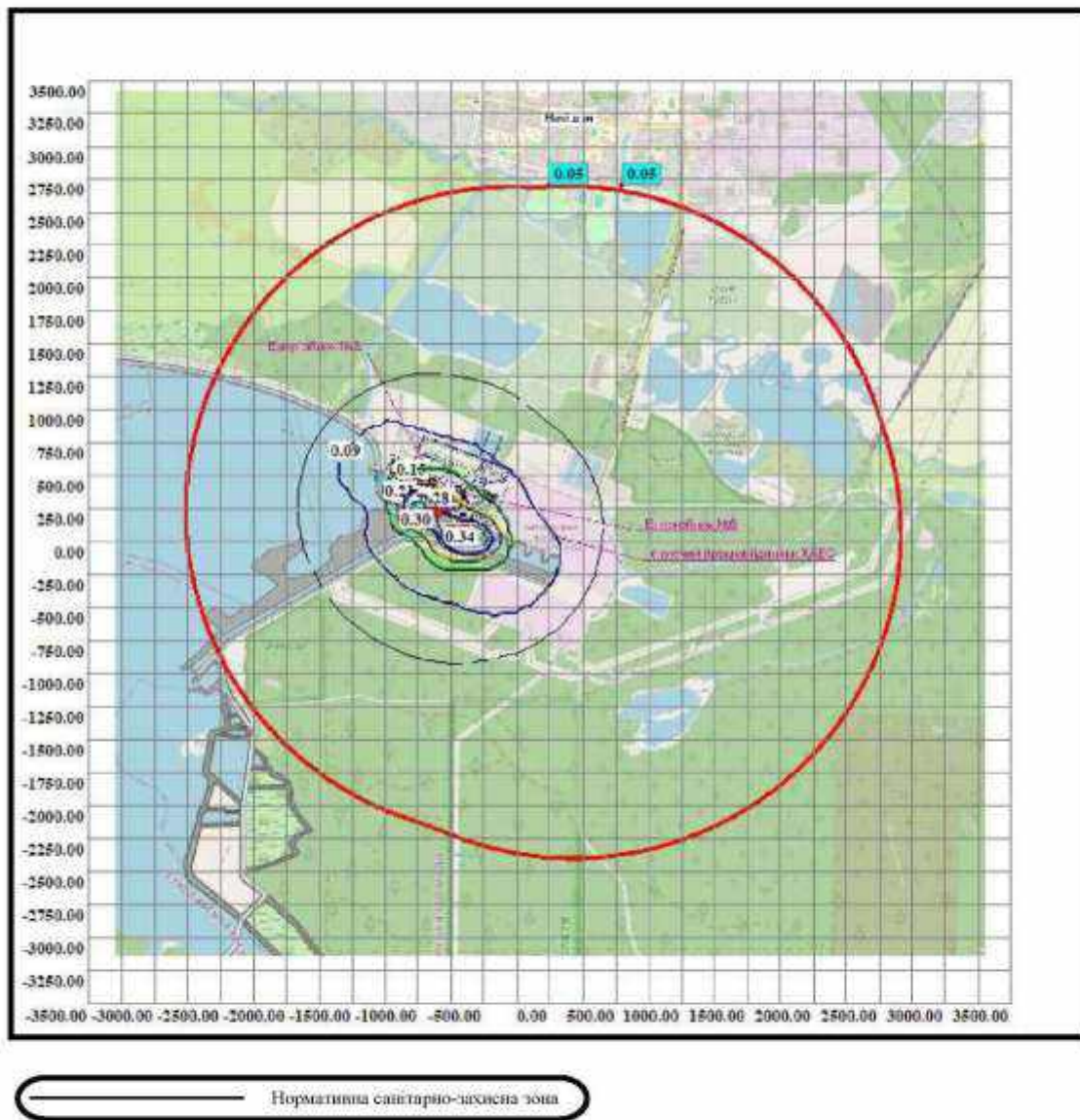
Антирад сферичний Карта-схема H=2.00 м
