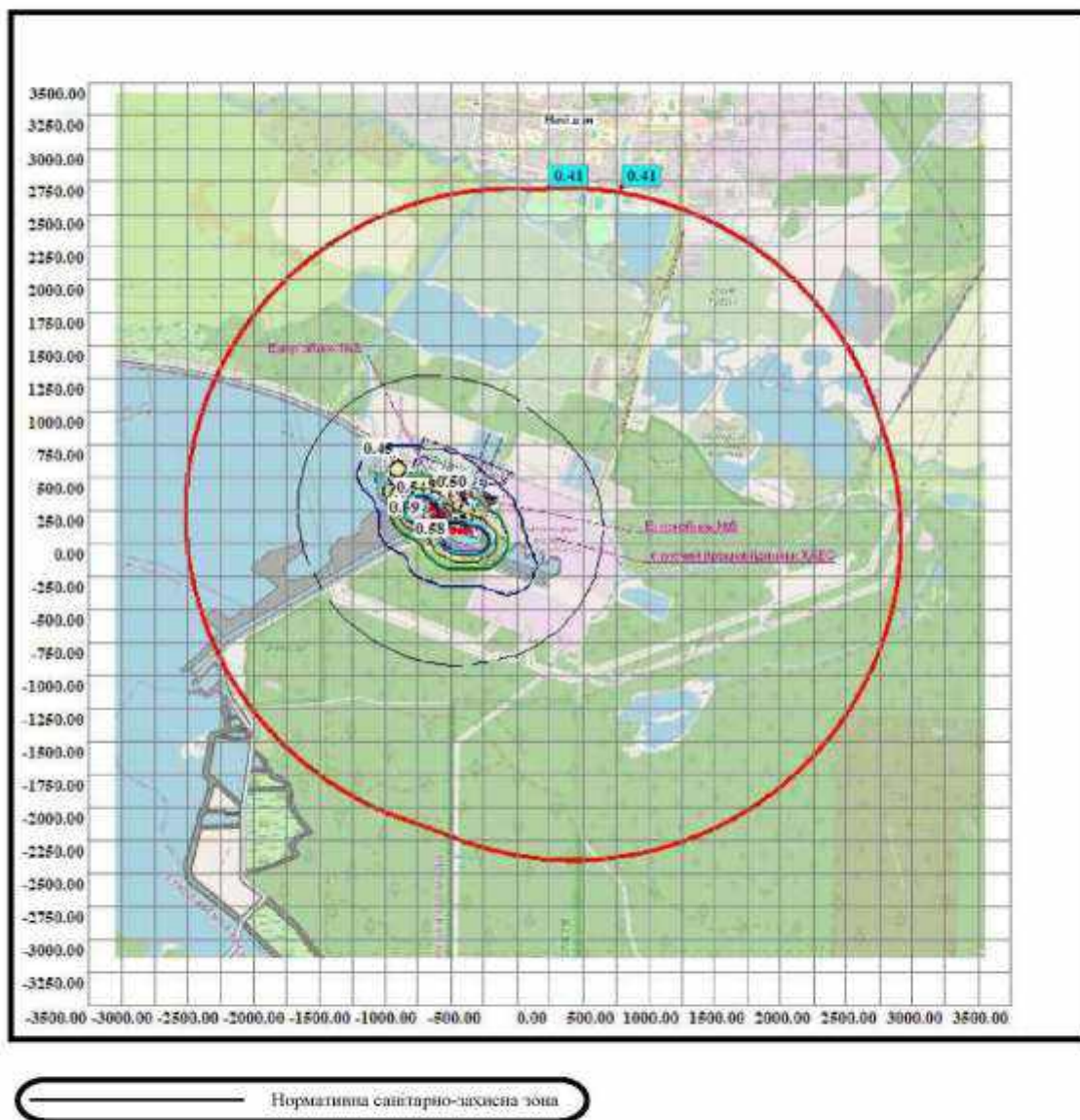
Вуглеводні границі с12-с19(розчинник РІК-26611 і ін.) Карта-схема Н=2,00 м
