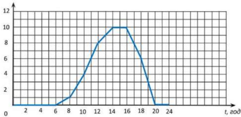
УФ – індекс
